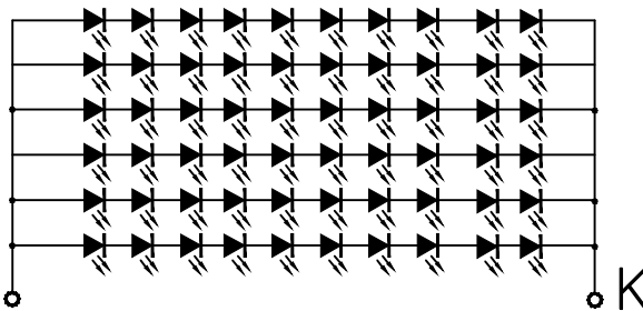
电路原理图: 10串X6并=60 LED
