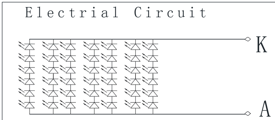
6 串 7 并 4 2 灯
